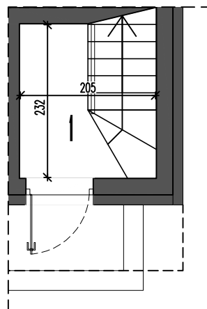
RZUT PARTERU
